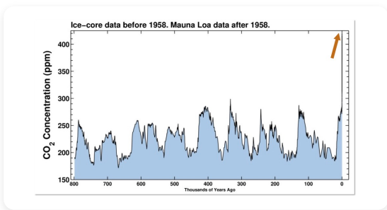
Figur: Keeling-kurvor med \text{CO}_2 -halt i atmosfären över 800.000 års respektive 300 års period (källa: https://keelingcurve.ucsd.edu/ ).
